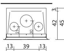
LUCE 62 PIANA - inserto a legna, con frontale in acciaio
