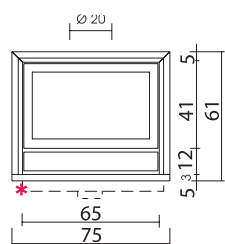
LUCE 62 PIANA - inserto a legna, con frontale in acciaio
