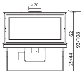
LUCE 54 PIANA - inserto a legna, con frontale in acciaio
