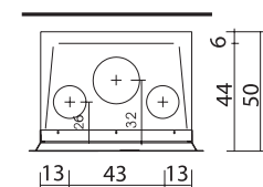
LUCE 62 PIANA - inserto a legna, con frontale in acciaio
