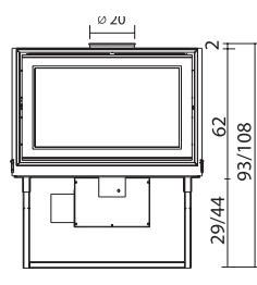
SCREEN 100 - focolare a legna, con frontale in vetro ceramico serigrafato
