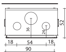
SCREEN 100 - focolare a legna, con frontale in vetro ceramico serigrafato
